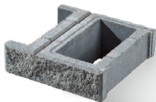
G1 Pustak podmurówkowy wys. 8 cm dł. 38 cm szer. 38 cm
